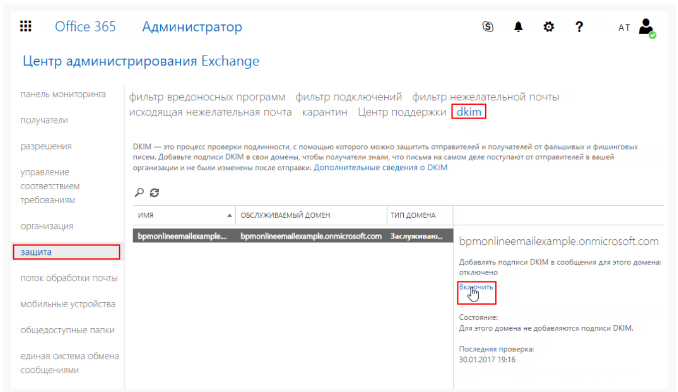
Рис. 3 — Включение DKIM для домена
