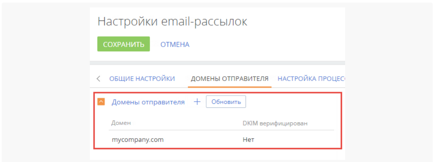
Рис. 2 — Вкладка [ Домены отправителя ]
