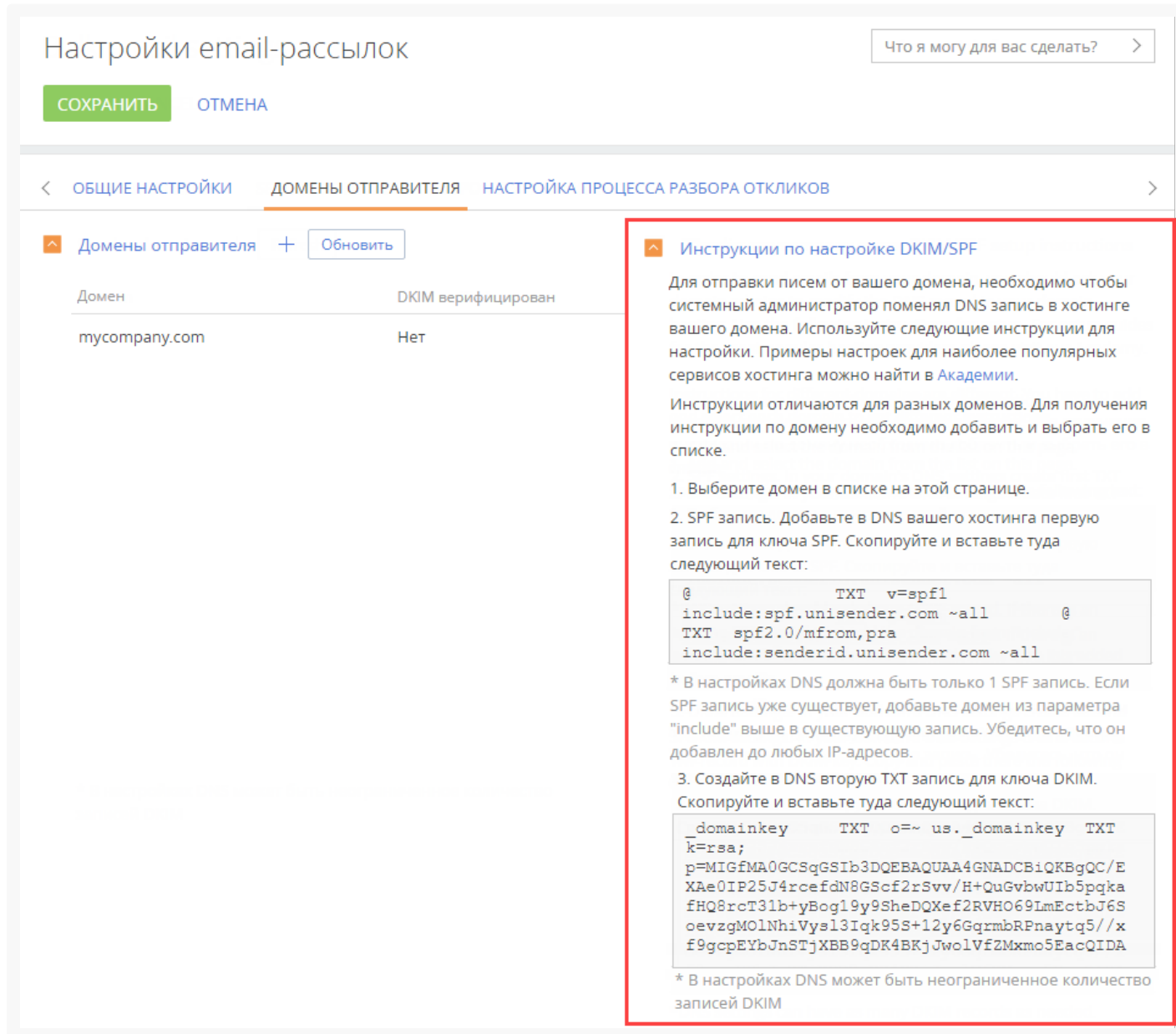
Рис. 3 — Ключи DKIM/SPF для указанного домена
