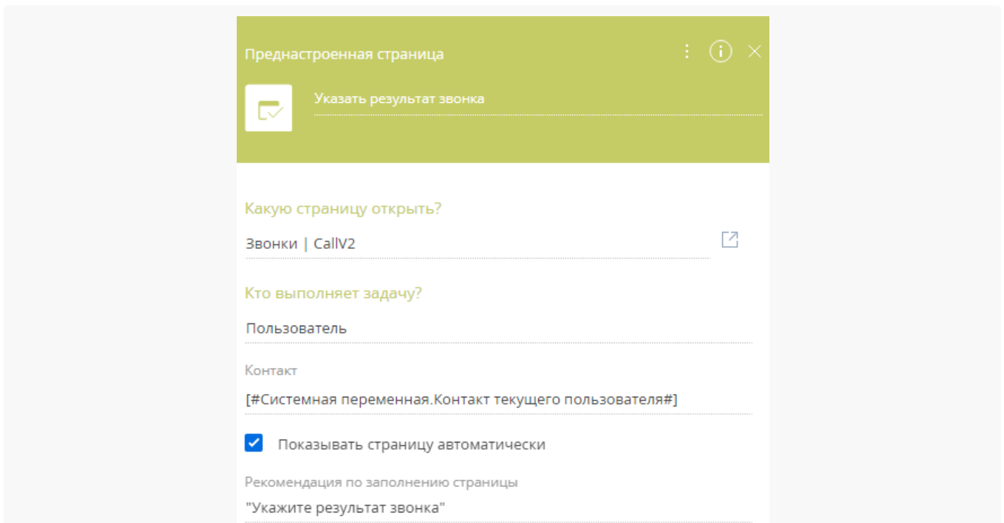
Рис. 3 — Пример панели настройки элемента [ Преднастроенная страница ]
