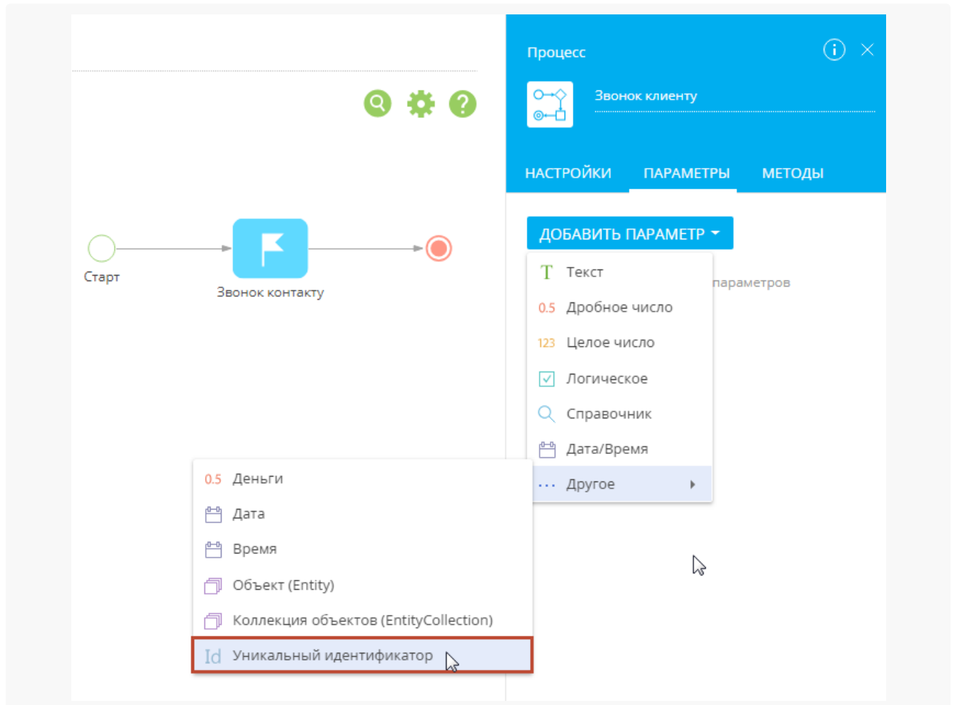
Рис. 2 — Добавление параметра в процесс
